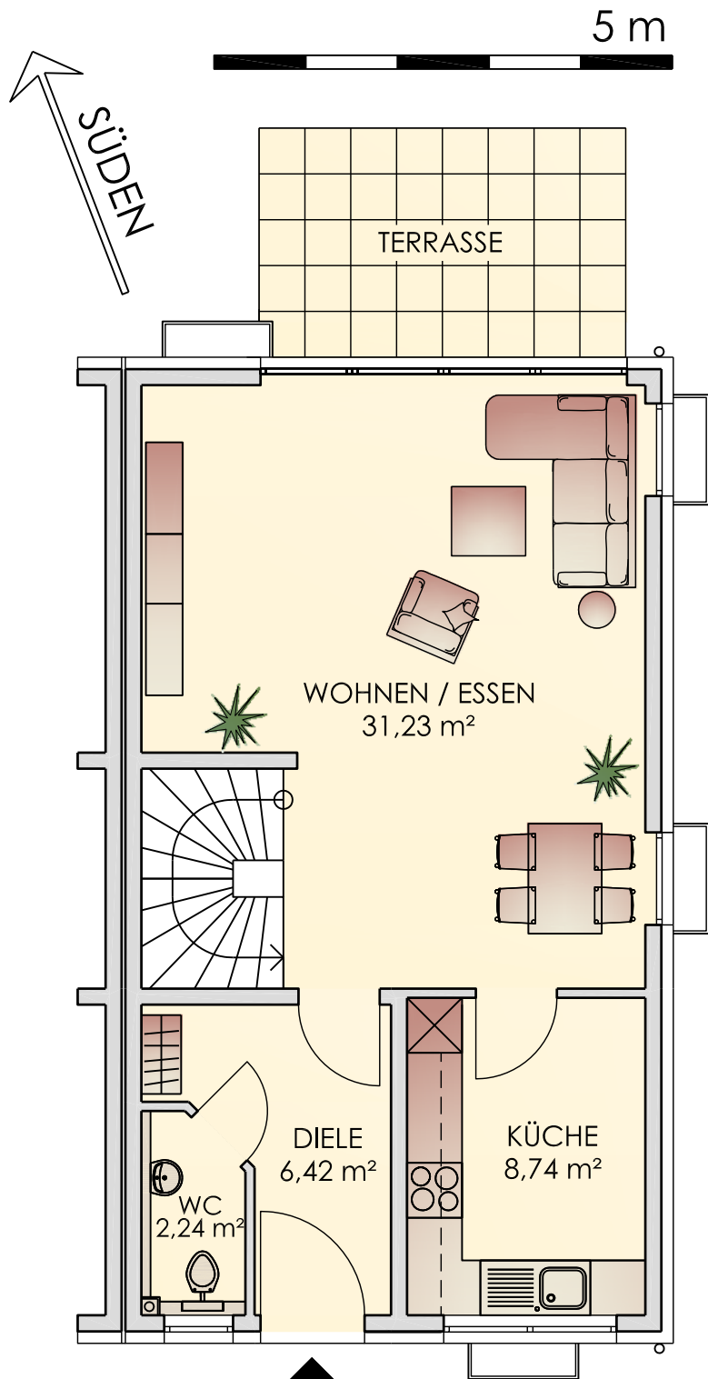
ERDGESCHOSS z. B. HAUS 2
