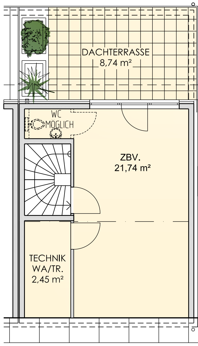
DACHGESCHOSS z. B. HAUS 2
