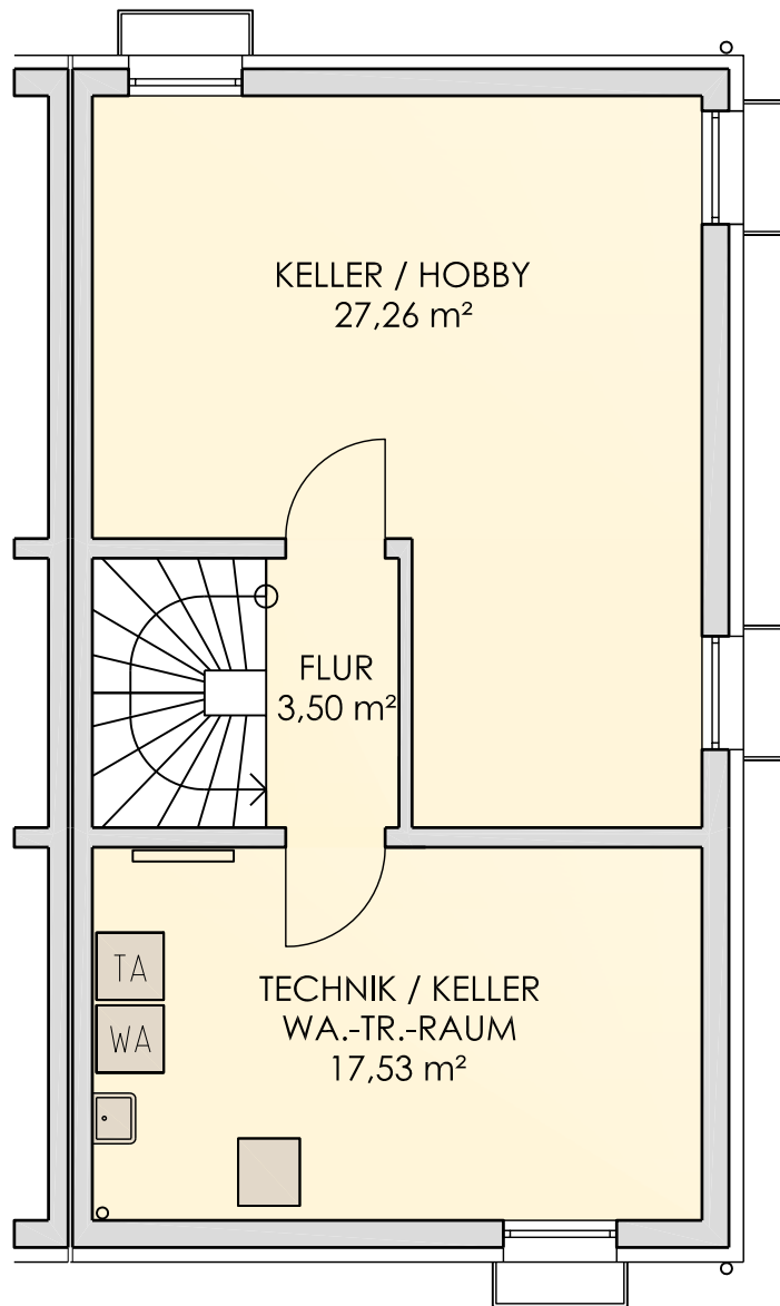
KELLERGESCHOSS z. B. HAUS 2
